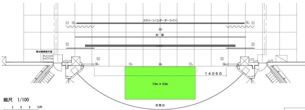
《輝きホール舞台図》
